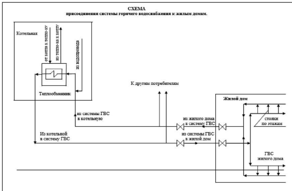
Рис.5. Схема присоединения систем горячего водоснабжения
